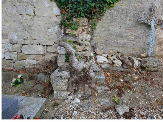
L'obtente et la destabilisation des maçonneries
